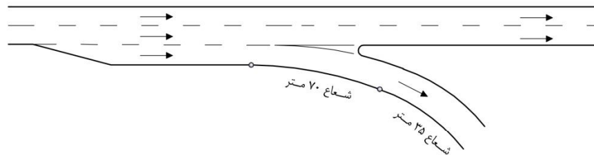
ب - قوس مرکب شعاع‌های ۳۵ متر و ۷۰ متر
