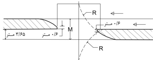
ب: M : ۵/۴ متر و بیشتر - لچکی طویل
