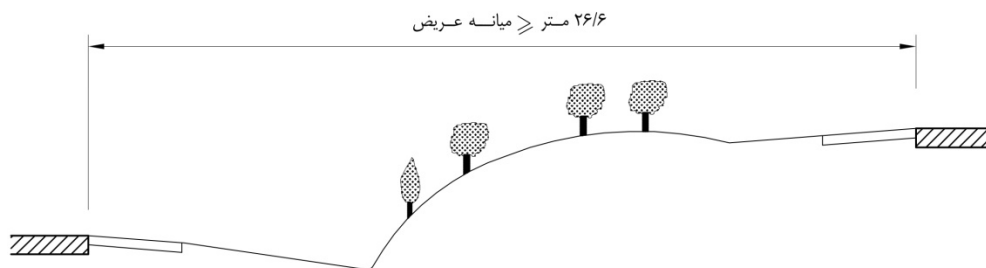
شکل ۶-۷- میانه بسیار عریض
