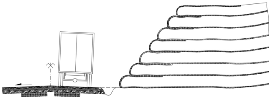
شکل ۶-۱۸ - خاک مسلح با پارچه‌گونه
