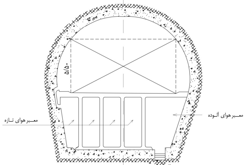
نمونه تهویه از پائین
