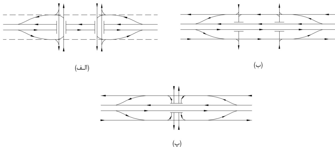
شکل ۹-۶- طرح‌های تبادلهای لوزوی به منظور کاهش برخوردهای ترافیکی
