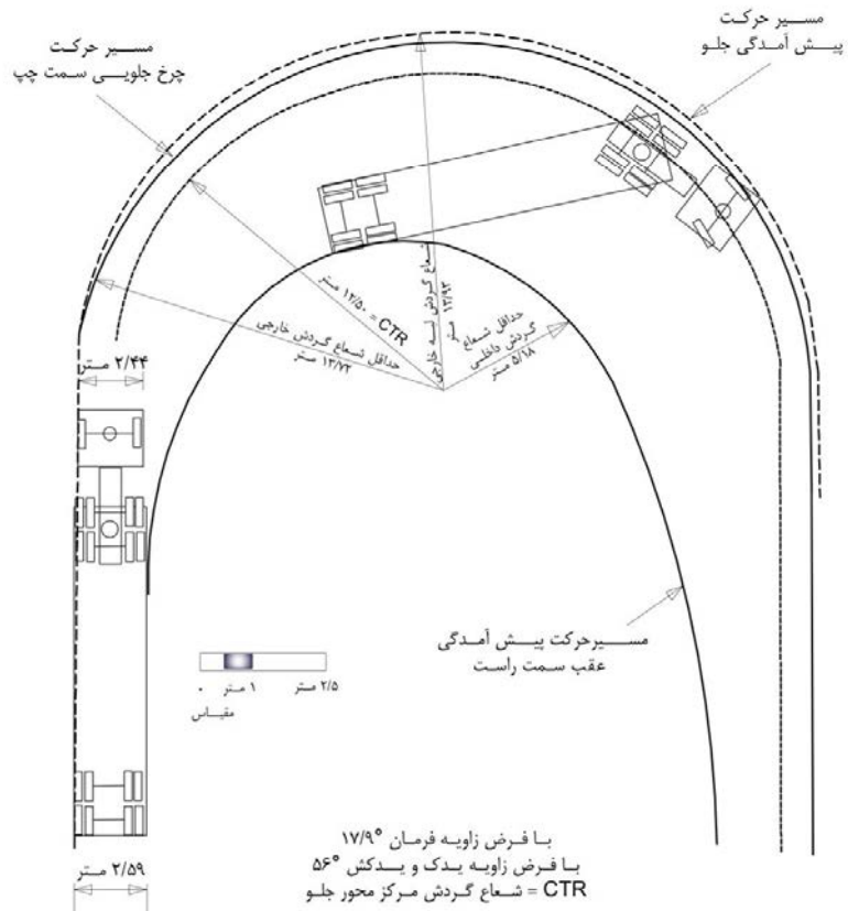
شکل ۴-۴ - مشخصات مسیر گردش خودروی طرح، کامیون نوع اول
