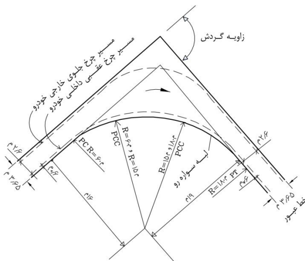
فوس مرکب سه مرکزی با شعاعهای ۶۰ - ۱۵ - ۱۸۰ متر و عقب نشینی ۴ متر
