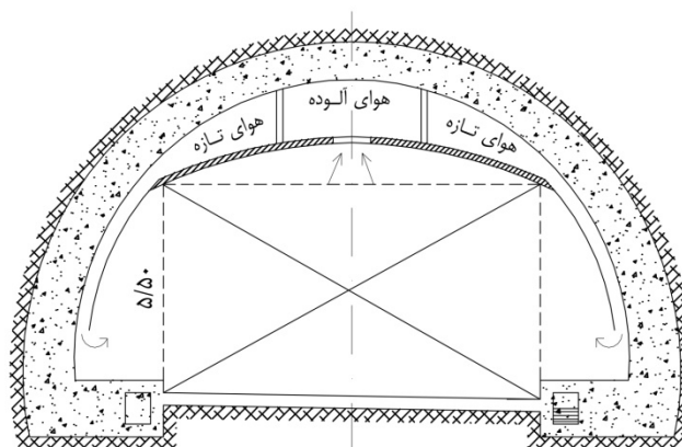
نمونه تهویه از بالا
