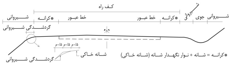
ب- جزئیات مربوط به کف راه دوخطه دو طرفه
