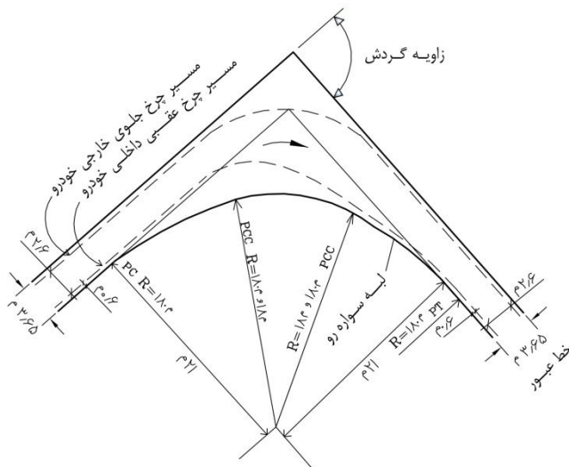
فوس مرکب سه مرکزی با شعاعهای ۱۸۰ - ۱۸ - ۱۸۰ متر و عقب نشینی ۳ متر
