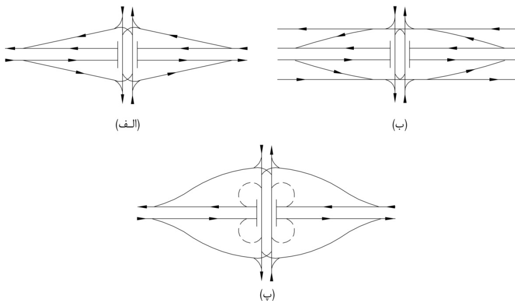
شکل ۹-۵- انواع ساده تبادلهای لوزوی
