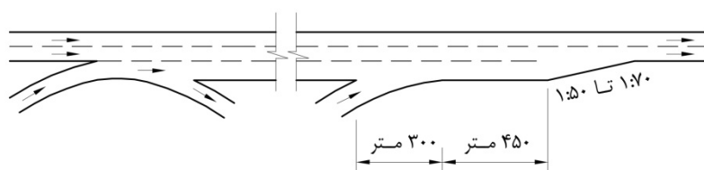
ث- حذف خط کمکی بعد از تبادل
